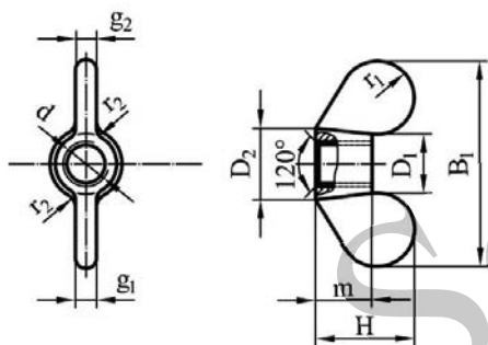
Piuliță fluture
