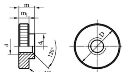
Piuliță striată
