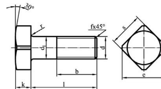
Șurub cu cap pătrat
