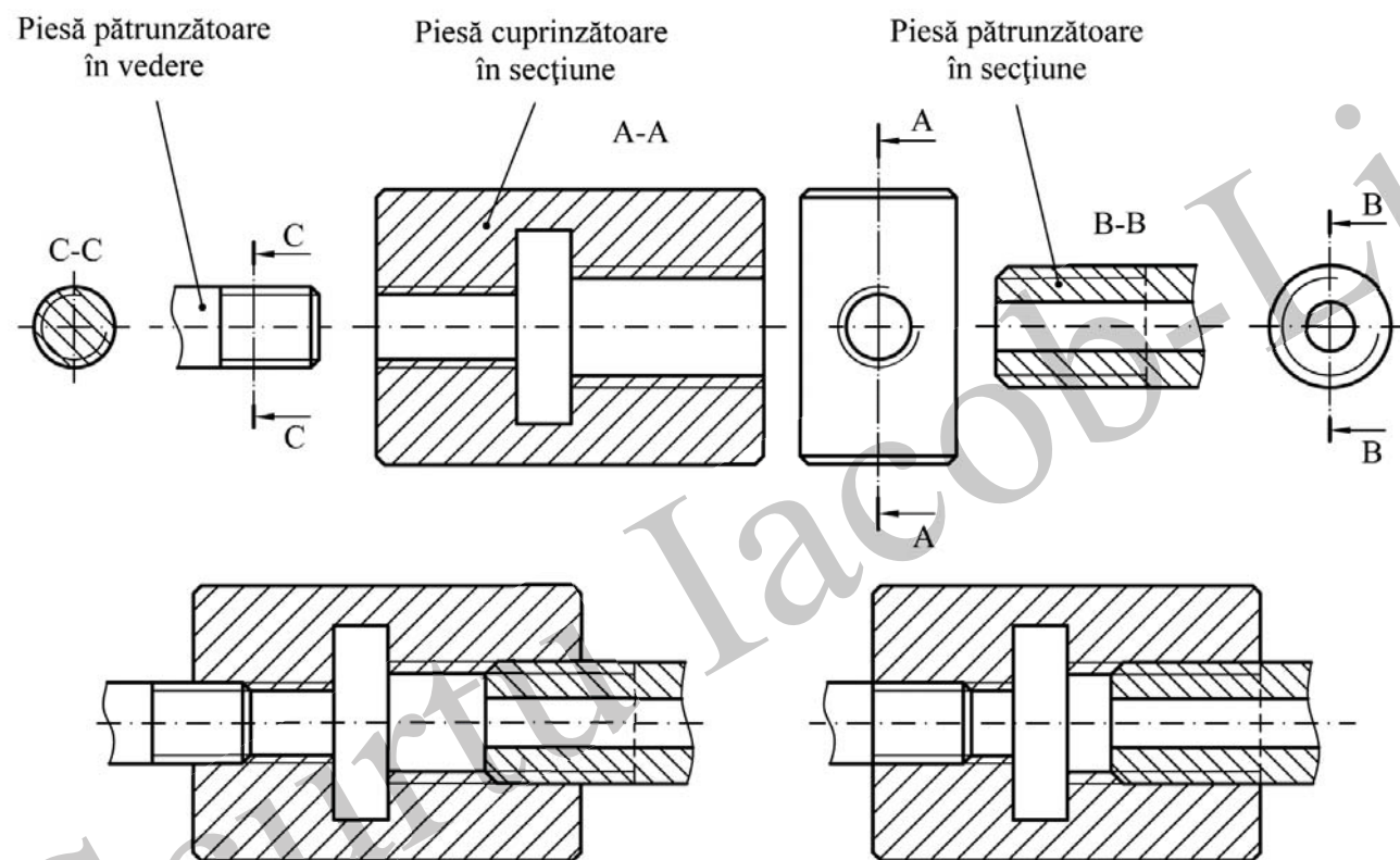
Asamblare prin filet, înfiletare incompletă
