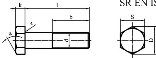
Șurub cu cap hexagonal
