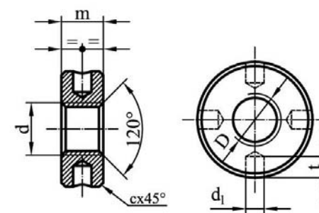
Piuliță rotundă cu găuri radiale
