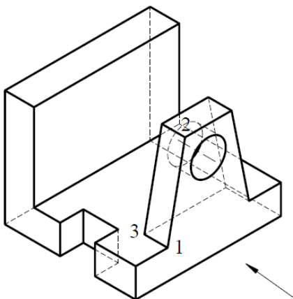
Fig. 1. Piesa reprezentată izometric- ap.2
