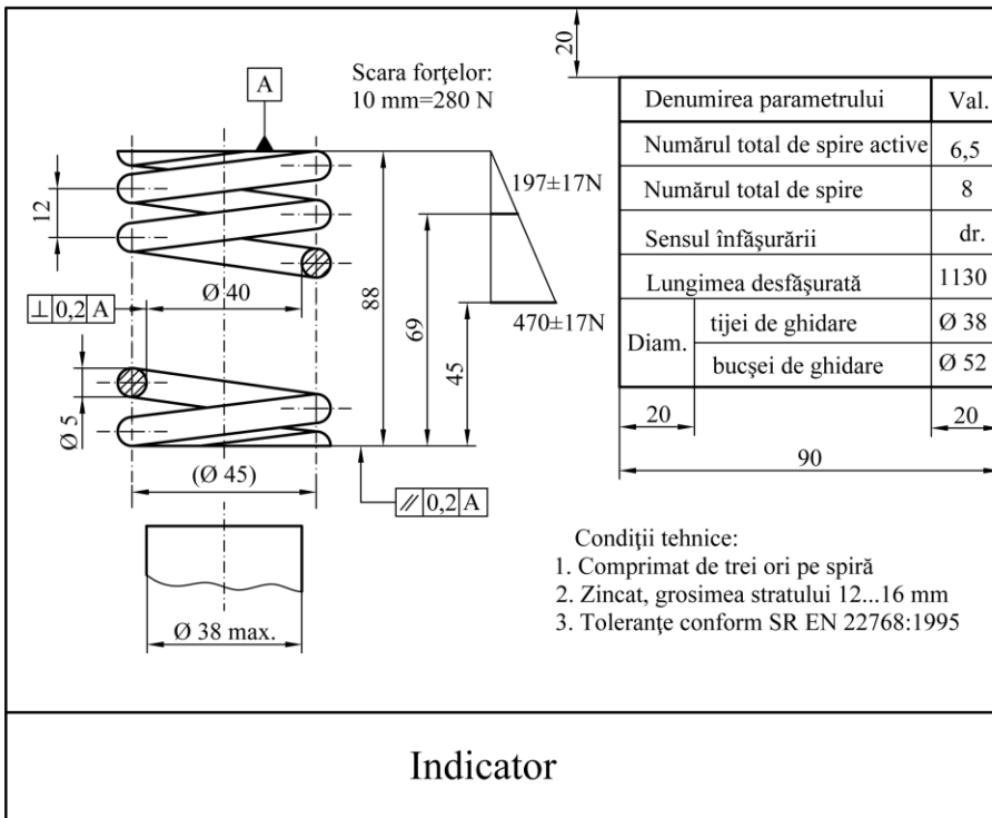
Fig.1 Arc elicoidal cilindric de compresiune - desen de execuție
