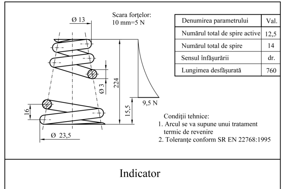
Fig. 2 Arc elicoidal conic - desen de execuție
