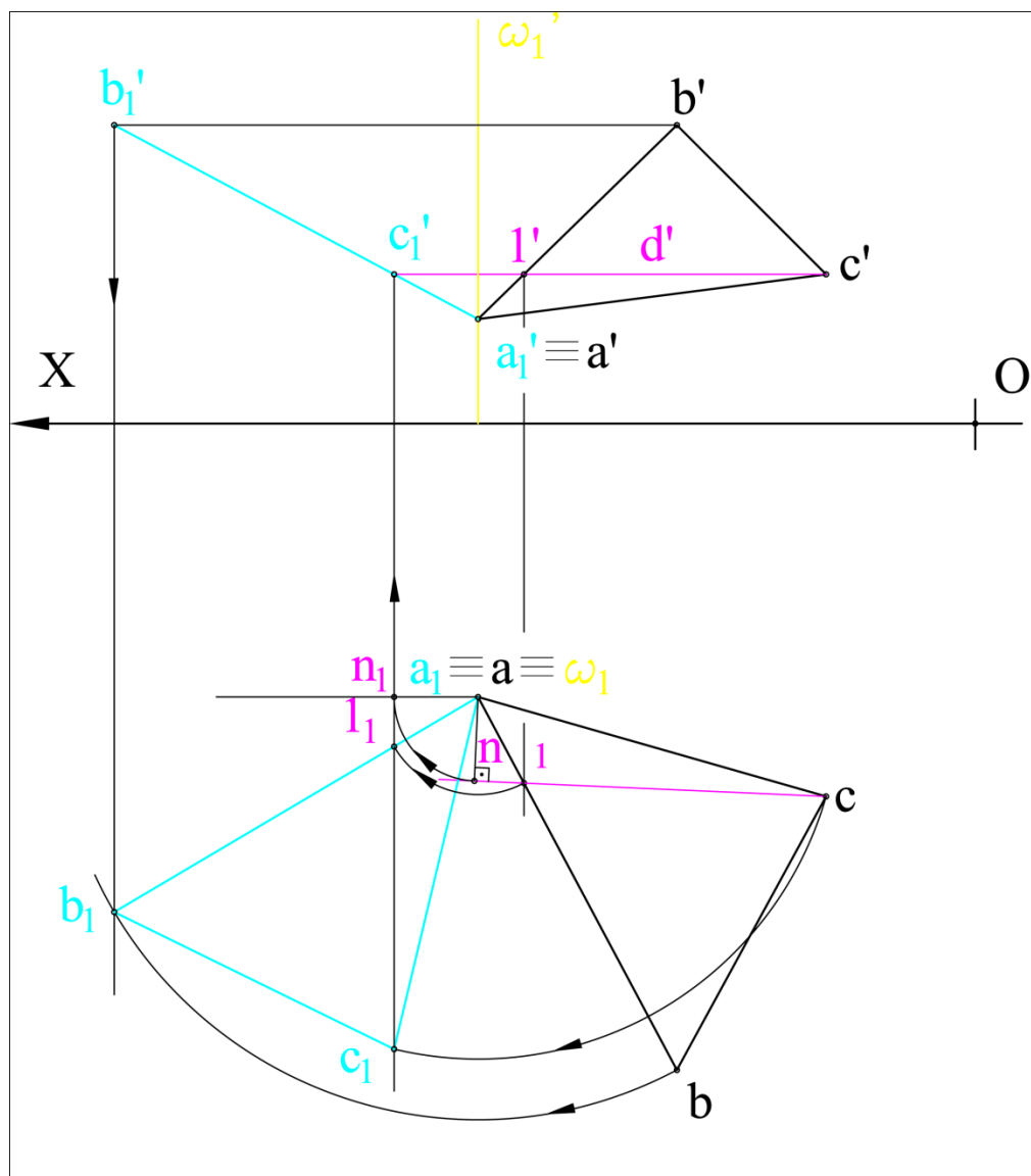
3. Rotația de front pentru placa triunghiulară –prima rotație
