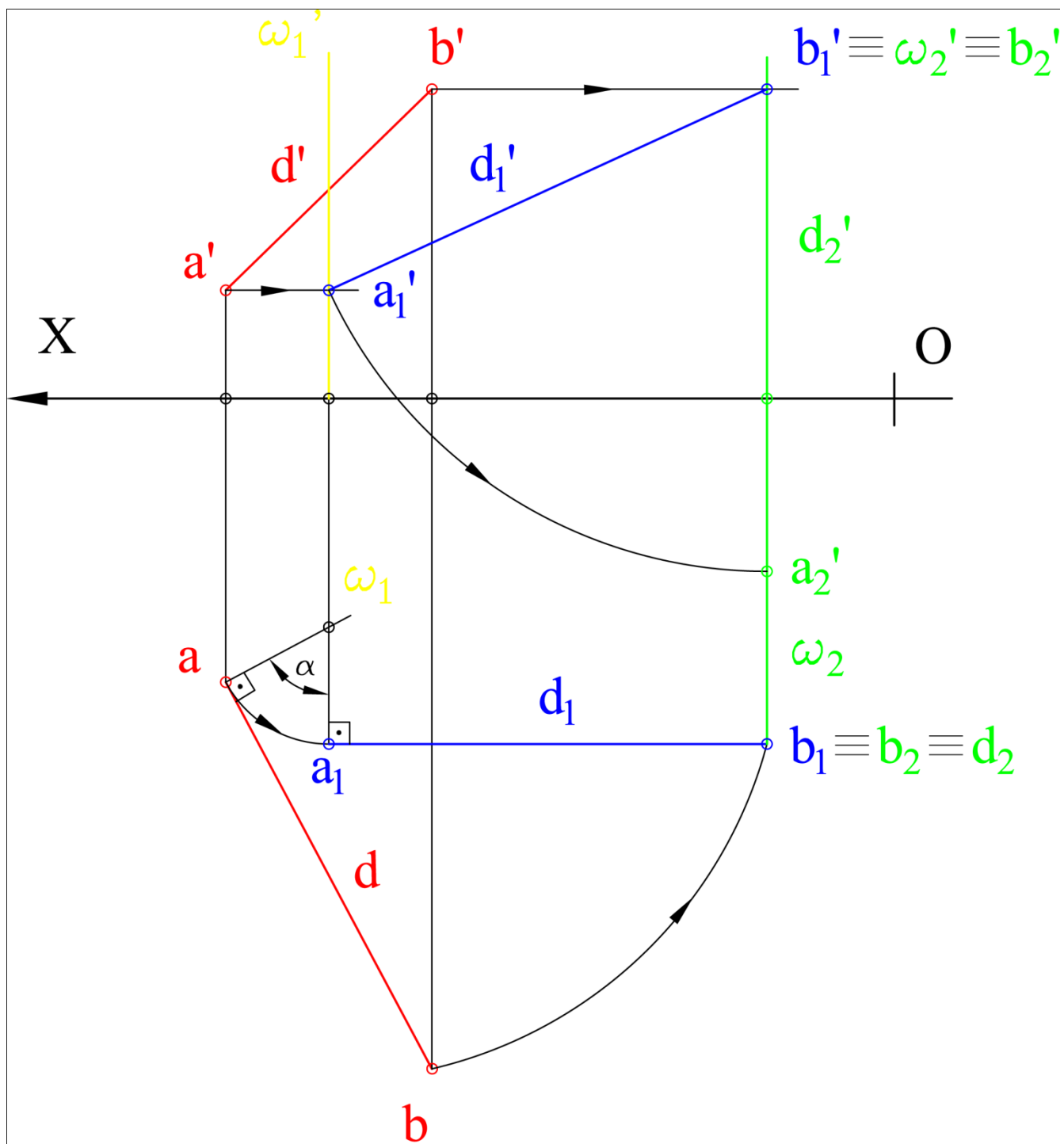
2.D2 –perpendiculara pe [H]
