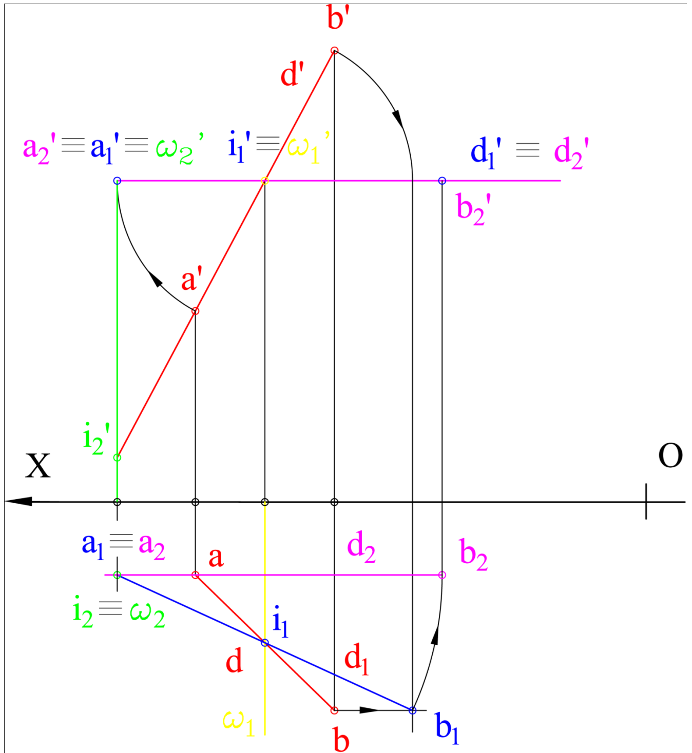
3.D2 –perpendiculara pe [L]
