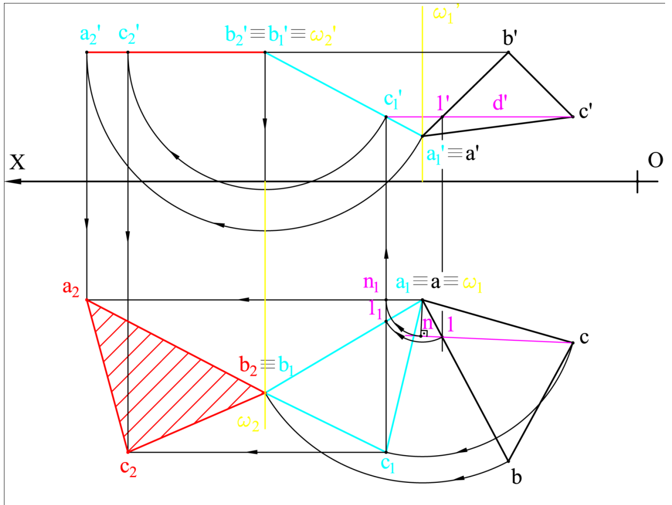
4. Adevarata mărime a triunghiului ABC prin dublă rotație
